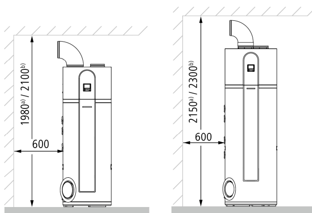
Fig. 2: Distances minimales (L et XL)
