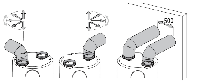
Fig. 11: Modes d'installation typiques
