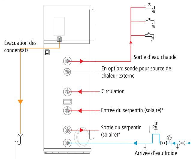
Fig. 5: Schéma de raccordement
