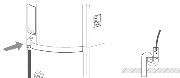
Fig. 8: Évacuation des condensats
