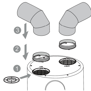
Fig. 11: Modes d'installation typiques
