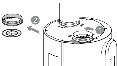
Fig. 13: Nettoyage du filtre à air
